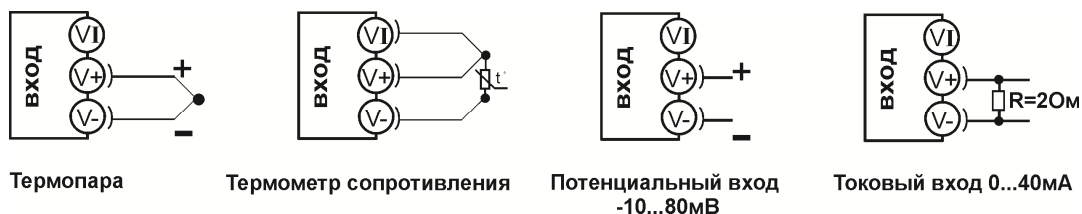
Рисунок 2. Схемы подключения датчиков
