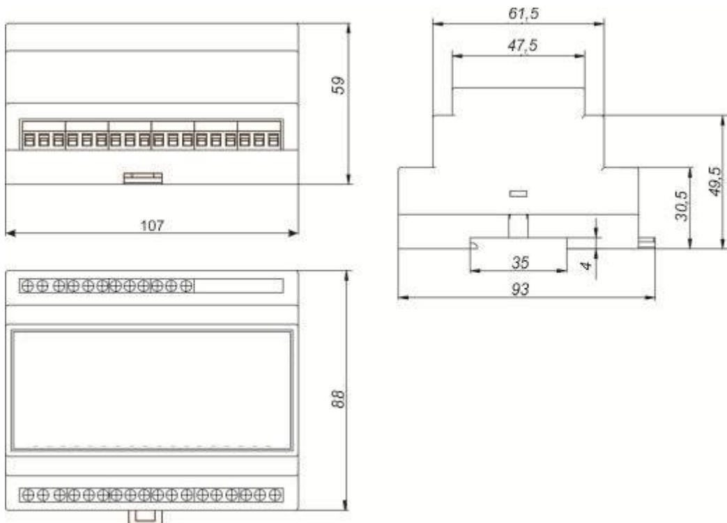
Рисунок 6 – Габаритные размеры блока измерения PB/12(24)УВ
